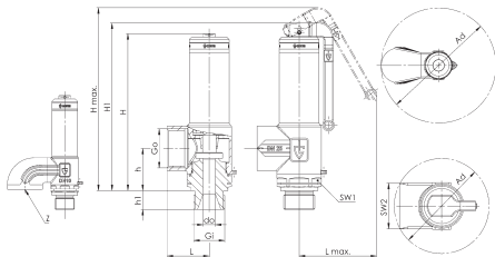
Общий вид клапана серии 2480
